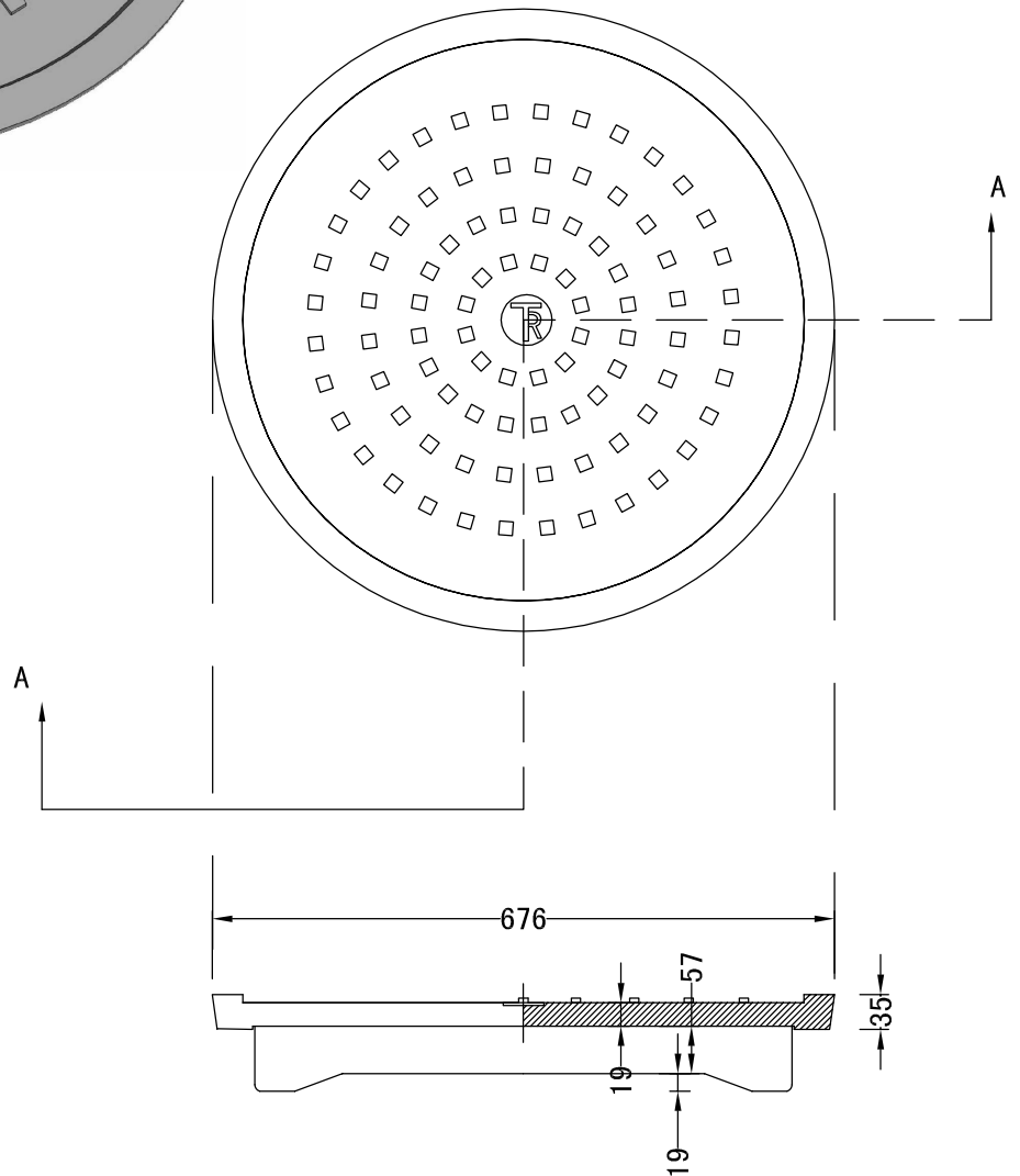
SECTION A-A
