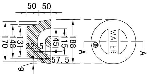
TYPE "A" VB LID
