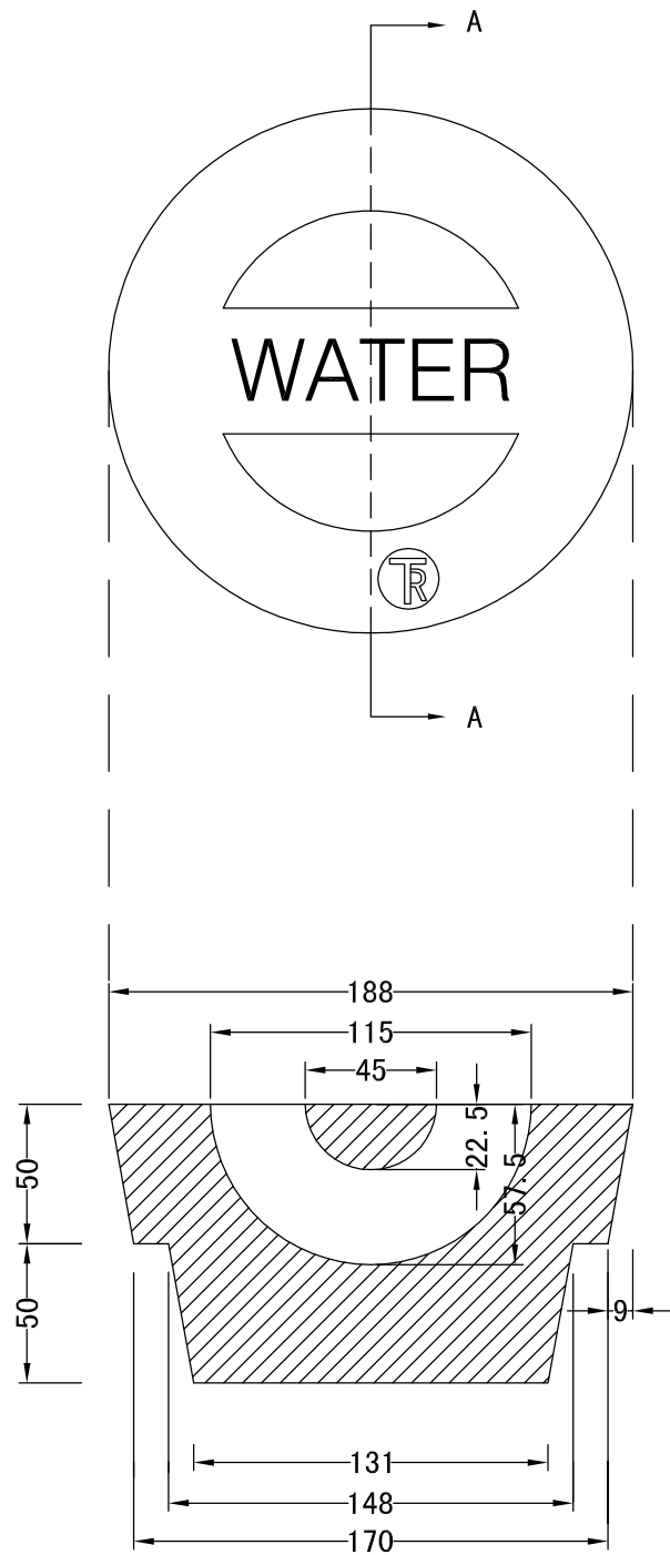
SECTION A-A
